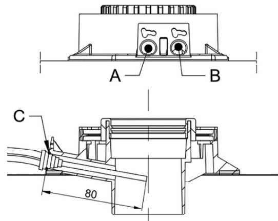
FIGURE 9-7 Orifice d'analyse de l'air nécessaire à la combustion et de la température
