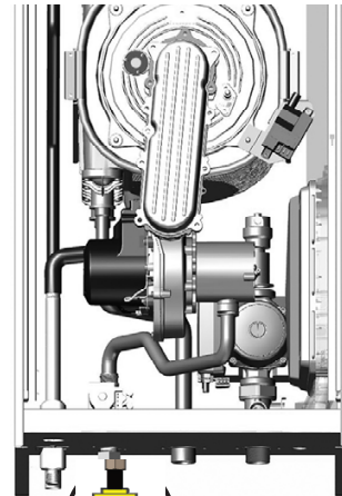
FIGURE 7-3 Robinet manuel principal d'approvisionnement en gaz à l'extérieur de la paroi de la chaudière
