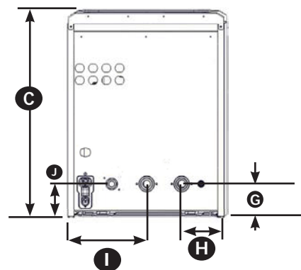
Vue de dessous Dimensions
