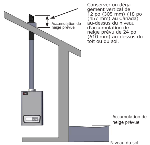
FIGURE 6-3 Évent coaxial pour installation sur le toit
