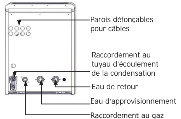
Vue de dessous Identification des raccordements
