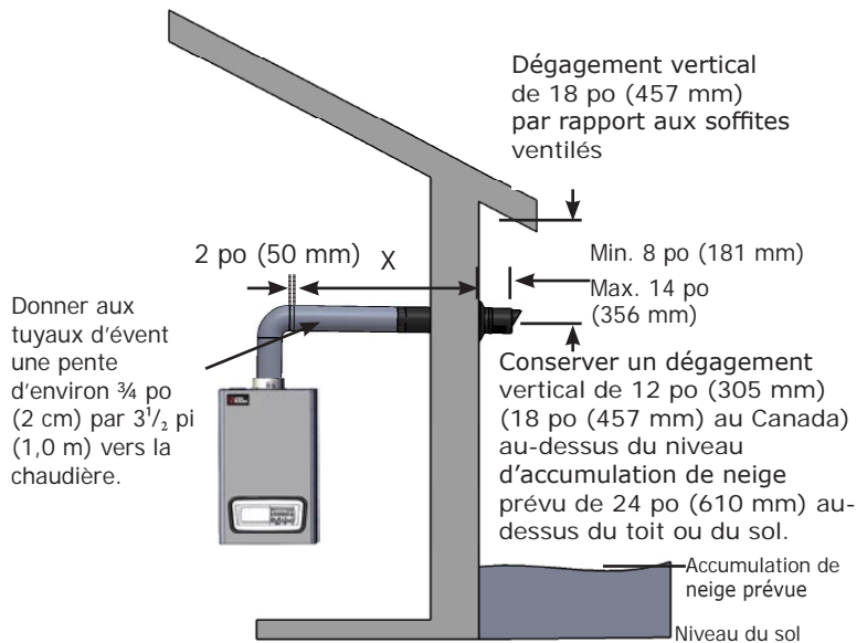
FIGURE 6-2 Évent coaxial pour mur latéral
