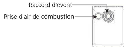
Vue de dessous Identification des raccordements
